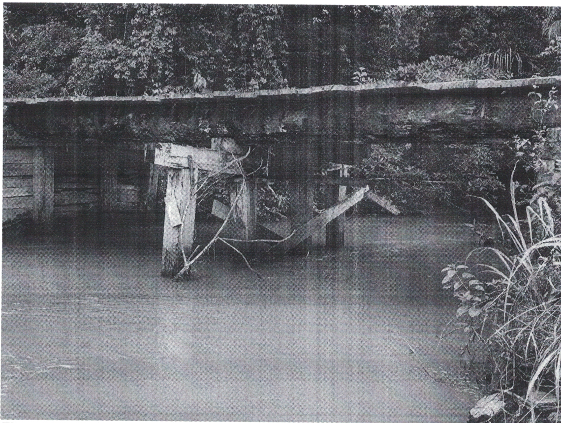
Figura 02. Ponte em madeira, localizada na Linha C-22. jan 2023.
